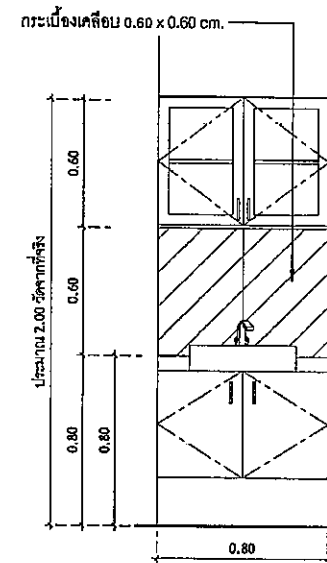
รูปด้าน CS-0.8/CF-0.8
