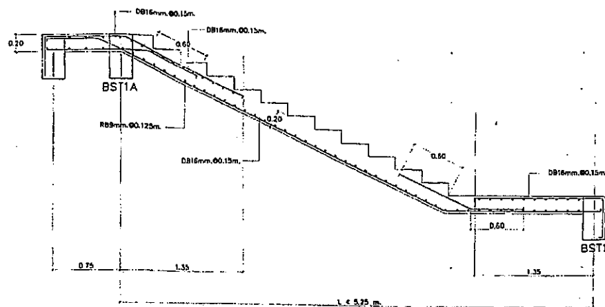
แปลนโครงสร้างบันได ST1 1:20
