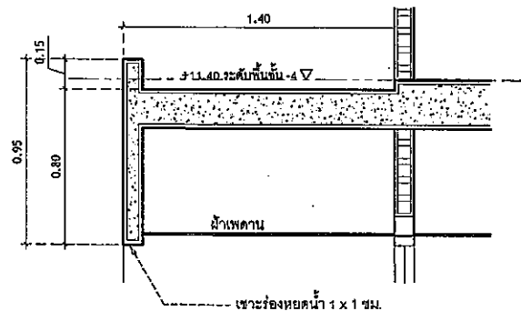
DT-6 ก๊วนสาด ค.ส.ล. 2 SCALE 1 : 25 (A3)
