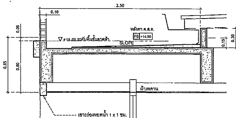
DT-5 หลังคา ค.ส.ล. 2 SCALE 1 : 25 (A3)
