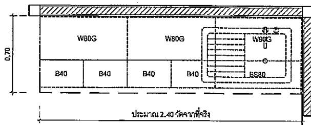
1 แปลน CS-2.4/CF-2.4 SCALE 1 : 25 (A3) ( ท้องถื่นเจ้าหน้าที ชั้น 1, 2, 3, 4 )
