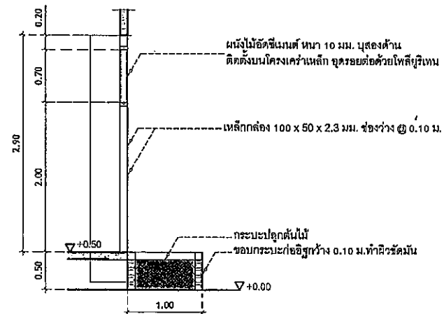
DT-1 รูปตัด แฉะระแนงกันสาด-2 SCALE 1 : 50 (A3)
