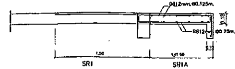
แบบขยายพื้น SR1,SR1A (CANTILIVER SLAB) SCALE 1:20
