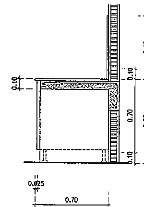
รูปตัด B CS-1.4/CF-1.4 SCALE 1 : 25 (A3)
