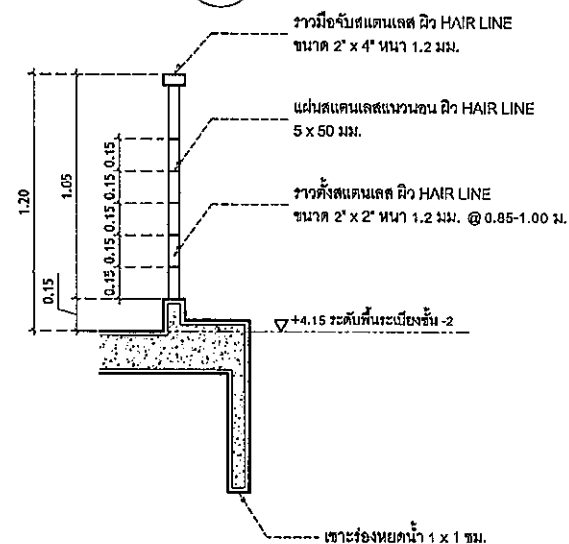
DT-7 แบบขยายราวกันตก SCALE 1 : 25 (A3)
