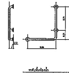
CT 791 (R) Multi-purpose hand rail ราวทรงตัวรูปตัวแอล ชนิดติดผนังด้านขวา
