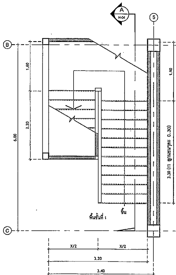
แปลนพื้นที่ - 1
