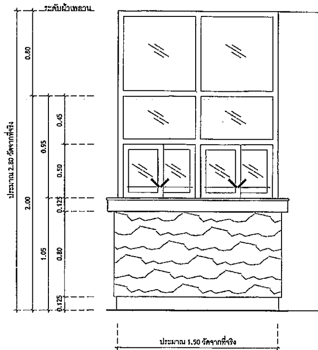
รูปด้าน B-1.4
