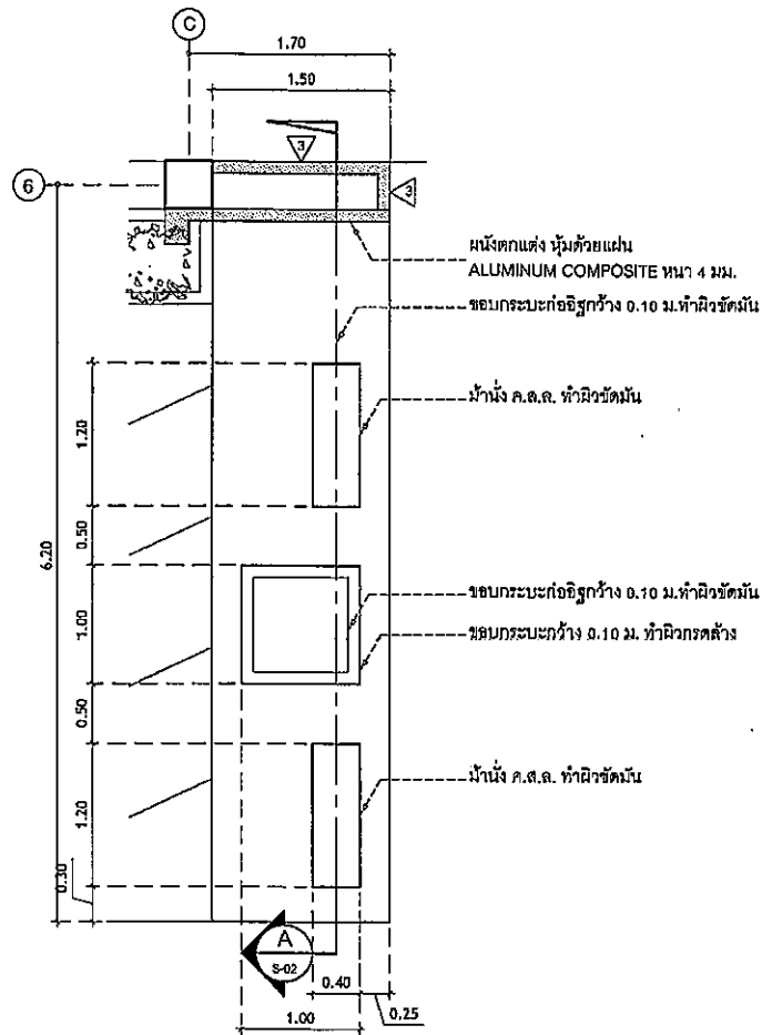
DT-2 แปลนกระเบื้องไม้, ผนัง SCALE 1 : 50 (A3)
