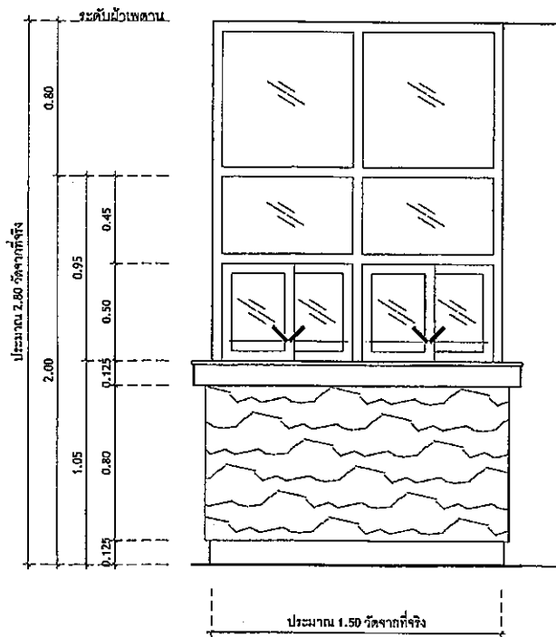
รูปด้าน B-1.5
