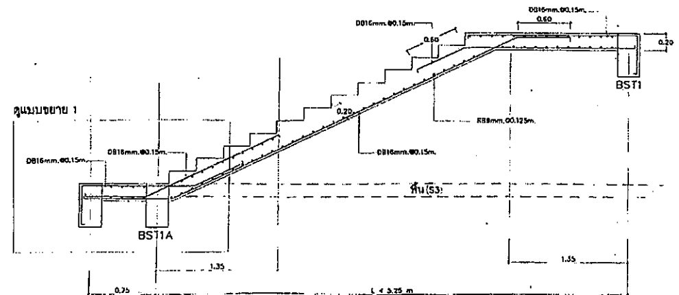
แปลนโครงสร้างบันได ST1 1:20
