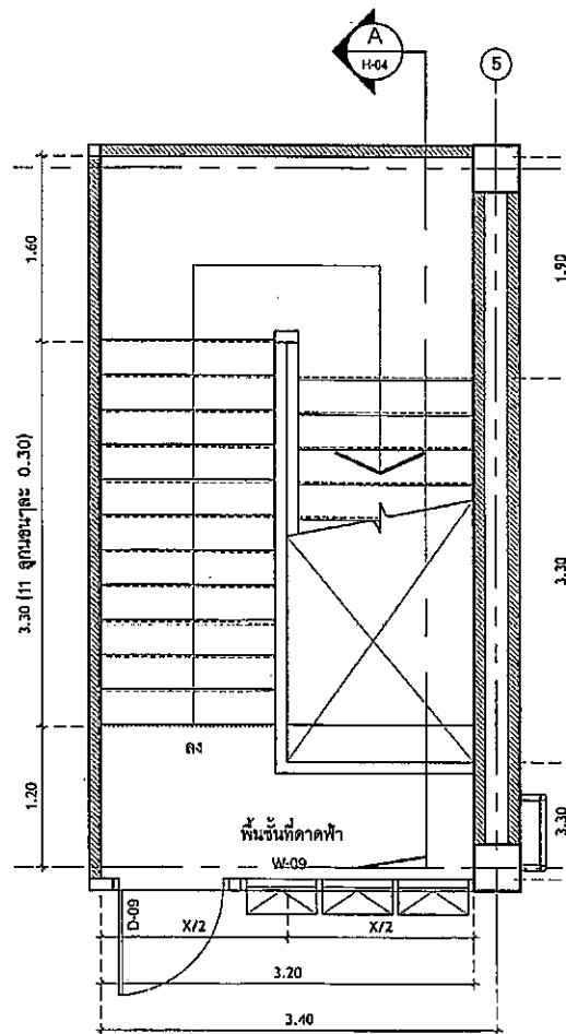
แปลนพื้นที่ลาดฟ้า
