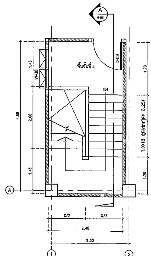
แปลนพื้นที่ - 4
