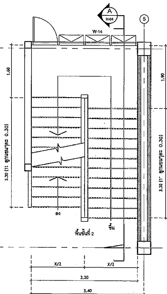
แปลนพื้นที่ - 2
