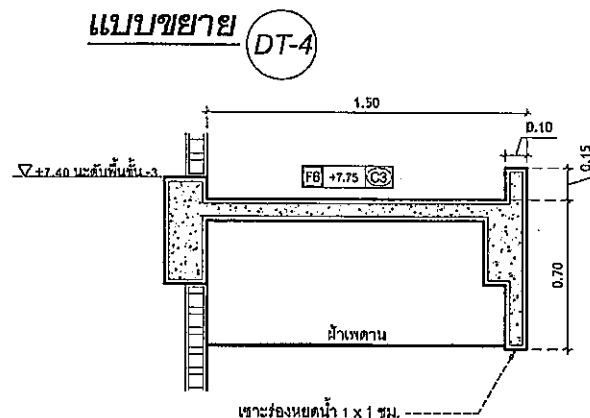
DT-4 กันสาด ค.ส.จ. 1 SCALE 1 : 25 (A3)
