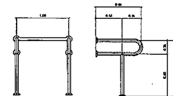
CT 795 Multi-purpose hand rail ราวทรงตัวสำหรับ อ่างล้างหน้า
