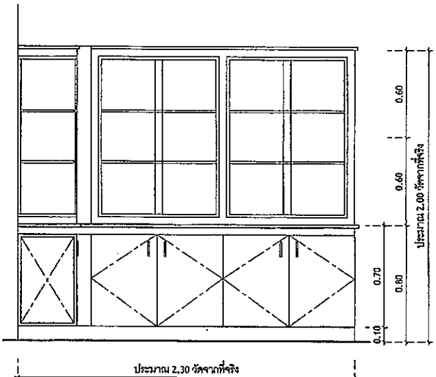
รูปด้าน CB-8 SCALE 1 : 25 (A3)
