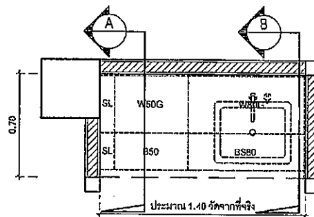
1 แปลน CS-1.4/CF-1.4 SCALE 1 : 25 (A3) ( ท้องถื่นเจ้าหน้าที ชั้น : ) ( ท้องถื่นเจ้าหน้าที , กิจกรรมกลุ่ม ชั้น 2 )
