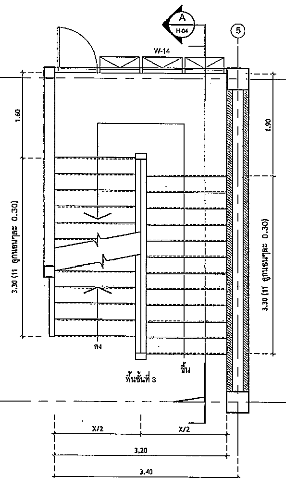
แปลนพื้นที่ - 3
