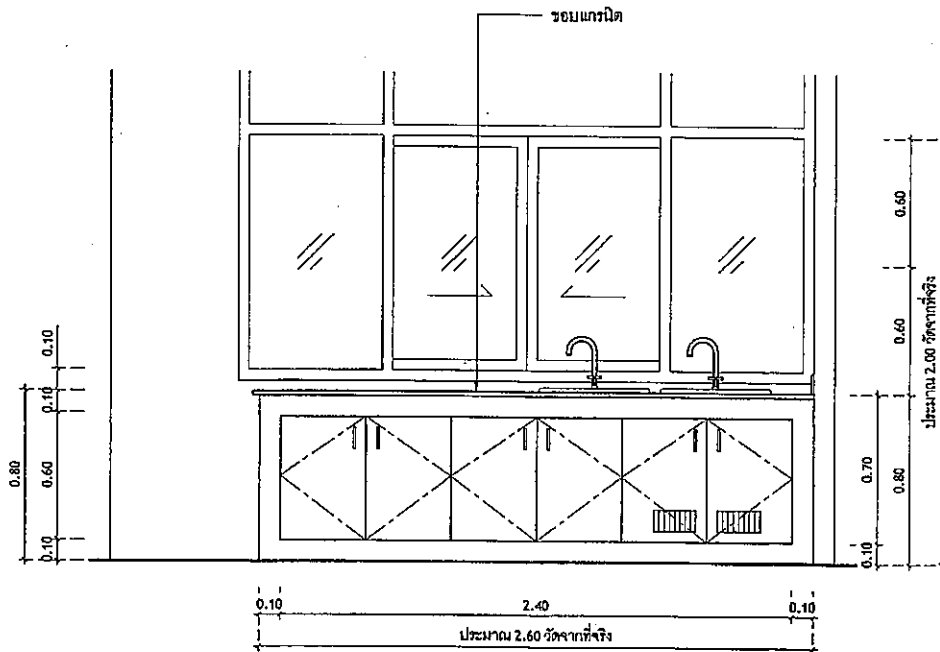
รูปด้าน CS-2.5
