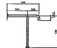
CT 793 Multi-purpose hand rail ราวทรงตัวรูปตัวที (T) สำหรับโถสุขภัณฑ์
