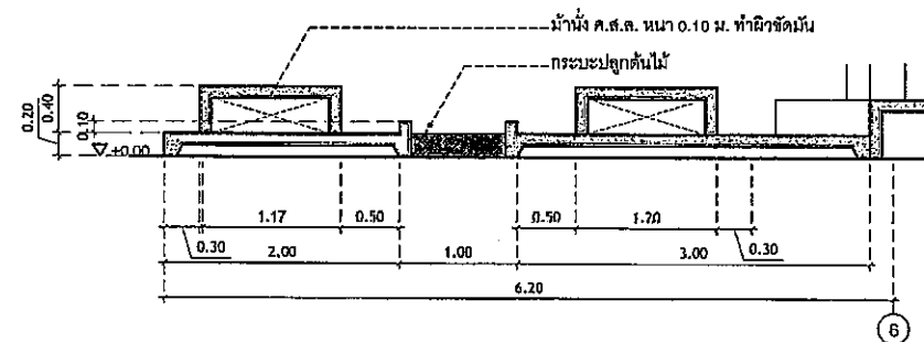
DT-2 รูปตัด A-A กระเบื้องไม้, ผนัง SCALE 1 : 50 (A3)
