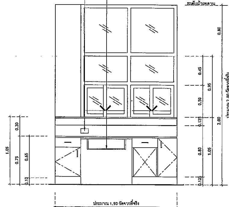
รูปด้าน B-1.4
